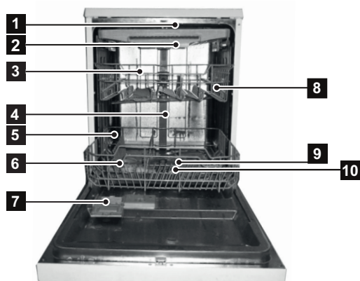
Čelní pohled
