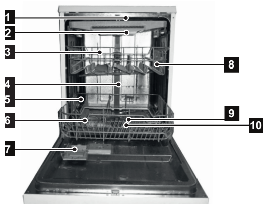
Pohľad zpredu
