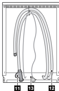
Zadní pohled
