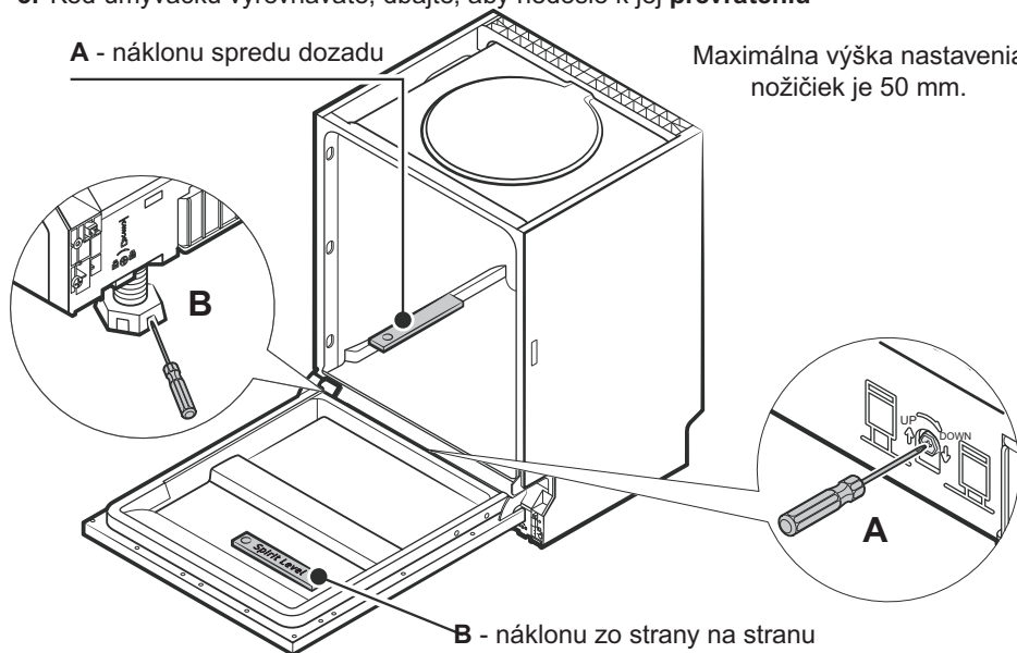
Obrázok 6 - vyrovnanie umývačky
